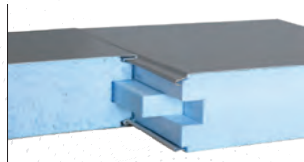
Giunto singola spina cortecce metalliche Single spine metallic facings joint
