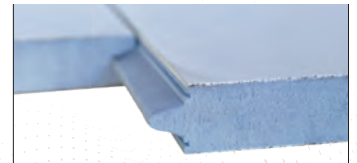
Giunto senza spina cortecce vetroresina No spine fiberglass facings joint
