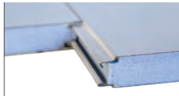
Giunto senza spina cortecce metalliche No spine metallic facings joint
