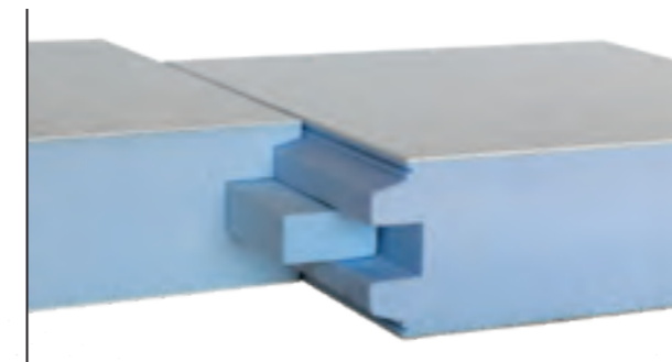
Giunto singola spina cortecce vetroresina Single spine metallic fiberglass joint
